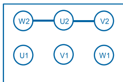
Y connection
