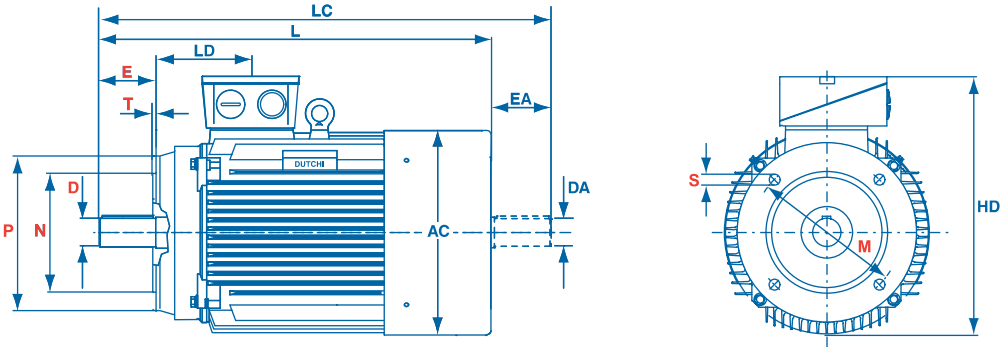
* DM1-HE 100 : L = 435 / DM1-HE 112 : L = 450
