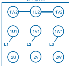
Y connection
