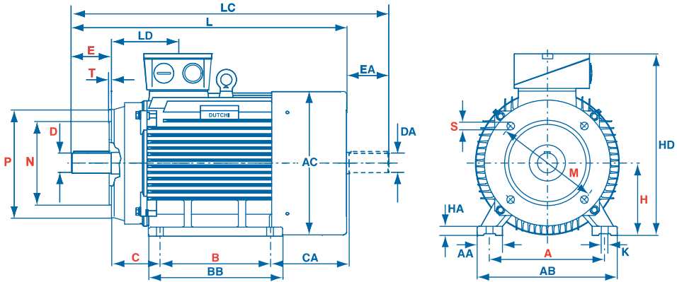
Flange measurements see DM1 80 - 160 : IM B14
