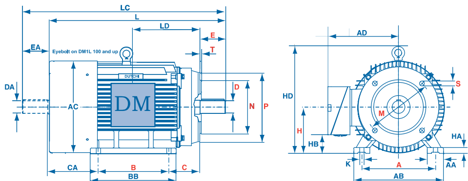
Flange measurements see DM1 80 - 160 : IM B14
